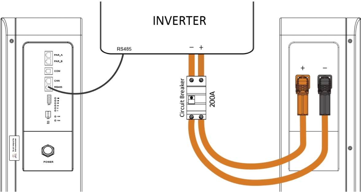
与逆变器连接示意图-推荐连接
