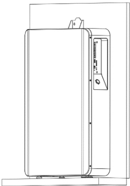
落地式
